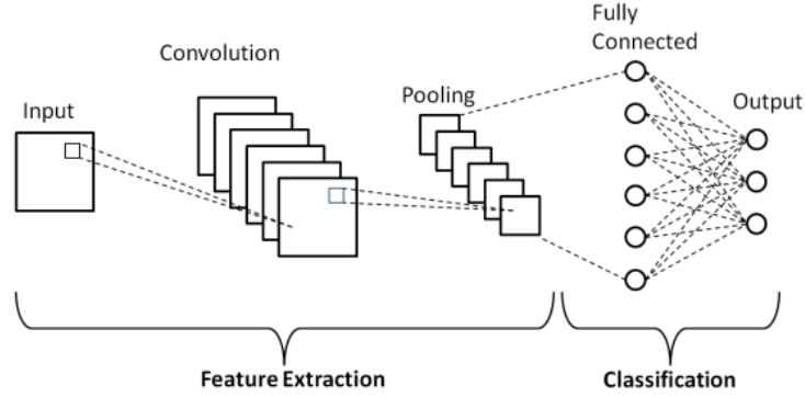
Fig. 1. : Estructura general de una Red Neuronal Convolucional y el concepto de convolución.
